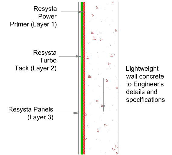
CROSS SECTION (Wall)
